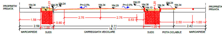
SEZIONE 25-25 - VIA GIACOMO MATTEOTTI - STATO DI PROGETTO
