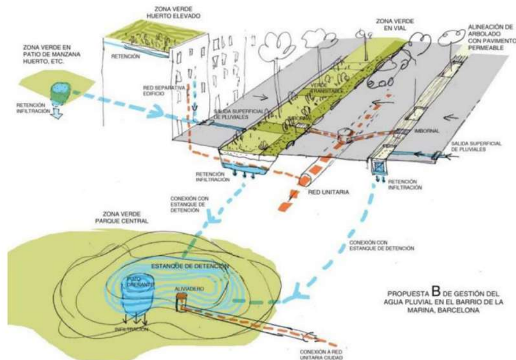
Diagram razlage delovanja SUDS
